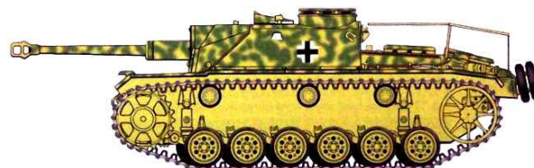
StuG III Ausf. G, Divisão Grossdeutschland, frente russa, maio de 1943. O capacete branco símbolo da Grossdeutschland é pintado na superestrutura. A pintura é em Dark Yellow e Dark Green.
